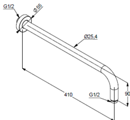
РАЗМЕРЫ
